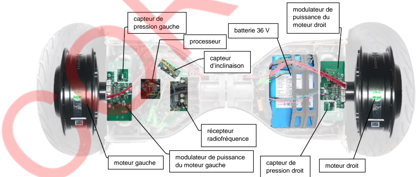
Figure 2 : vue interne de l'overboard Xenox
