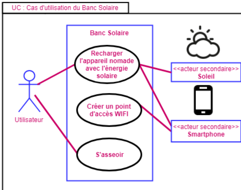
Document 1 : Diagramme des cas d'utilisation
